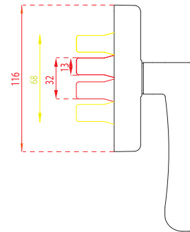
4021 / Normal Fork 4021 / Uzun Dil
