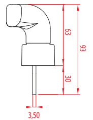
4022 / Double Fork 4022 / Çift Dil
