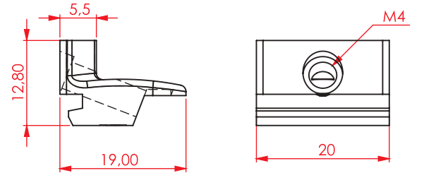
Fixed Striker B Sabit Karşılık B Item Code 824010
