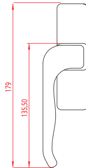
4020 / Short Fork 4020 / Kısa Dil
